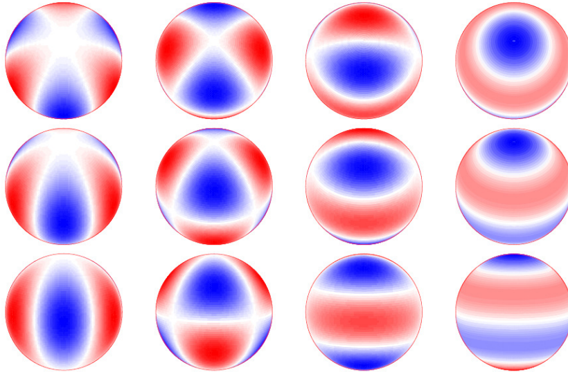
Figura 1: Diferentes modos presentes en una estrella pulsante.
